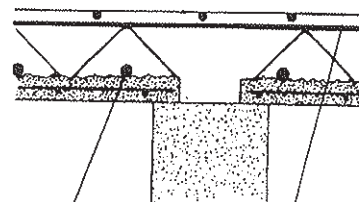
Krydsarmering Indspændingsnet
